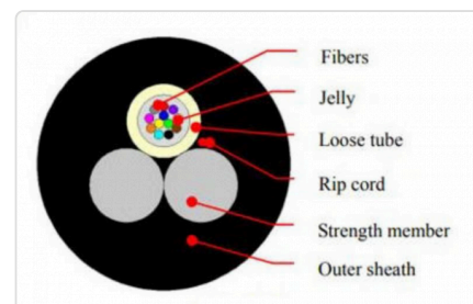
Mặt cắt cáp ASU KCO (ảnh hăng)
