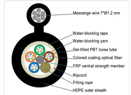
Cấu trúc cáp số 8 GYTC8S KCO (ảnh hăng)
